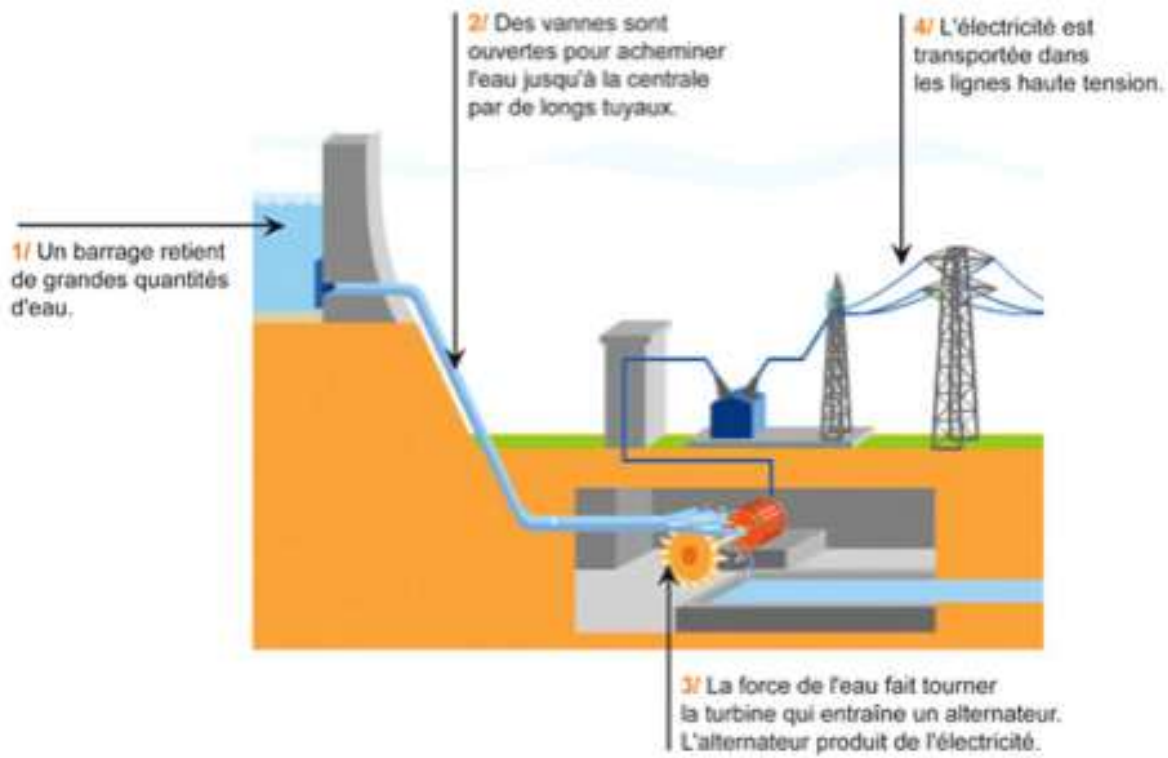
► Le fonctionnement d'une centrale hydraulique de haute chute © EDF
